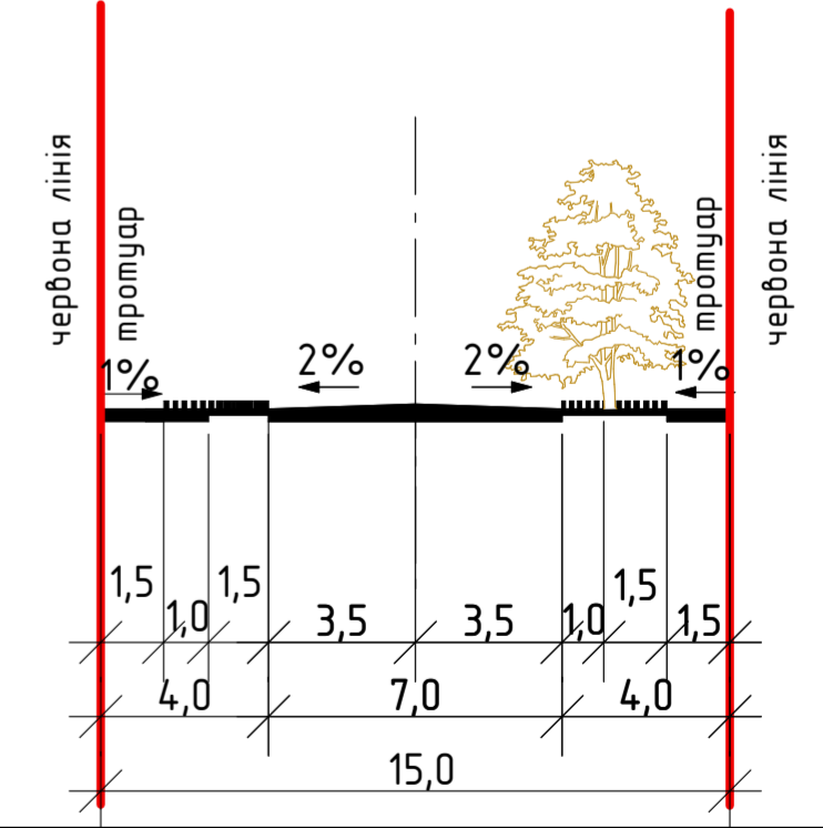
Креслення поперечних профілів вулиць М 1:500 Житлові вулиці вул. Хмельницького
